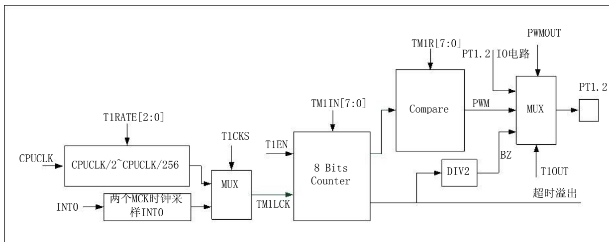
图10 定时/计数器 1模块的功能框图
