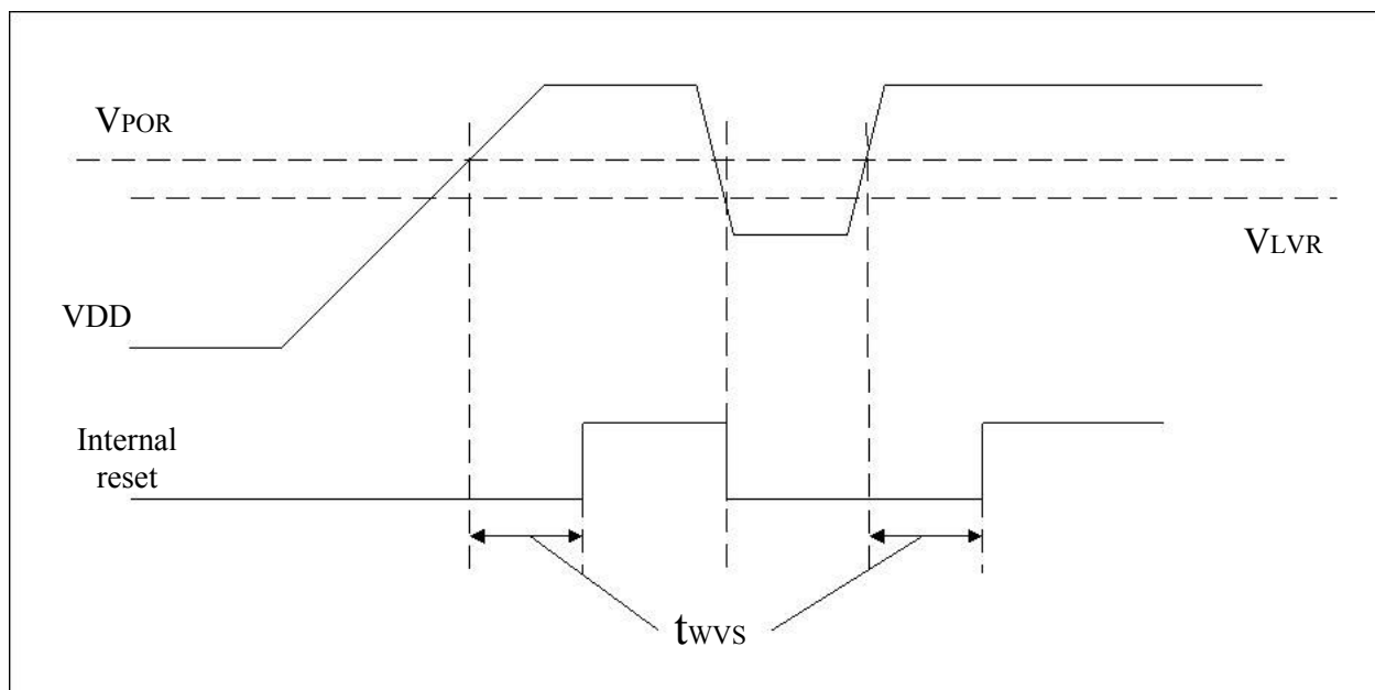
图7 上电复位电路示例及上电过程
