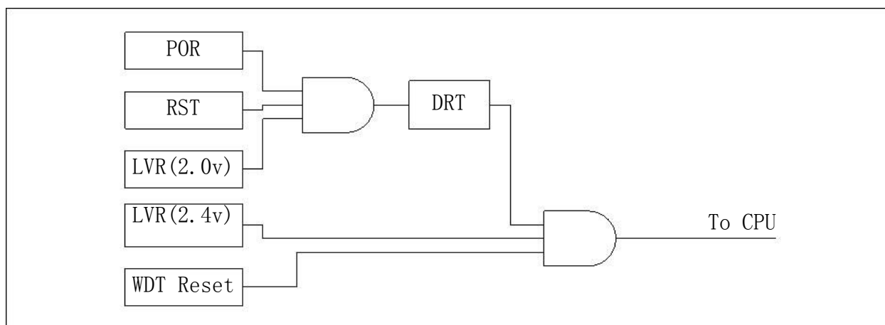
图6 复位电路原理图
