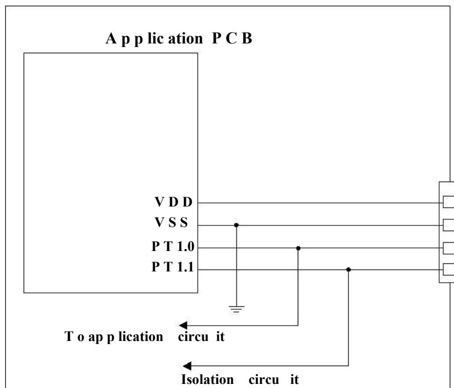
图12 烧写器接口图
