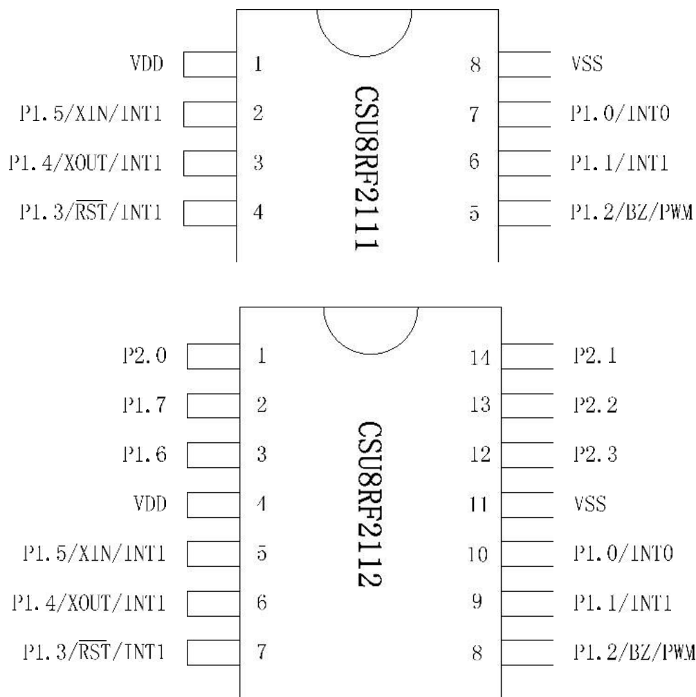
图1 8/14-pin配置图
