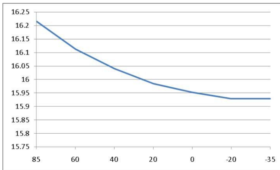
图 12内部晶振频率随温度变化曲线
