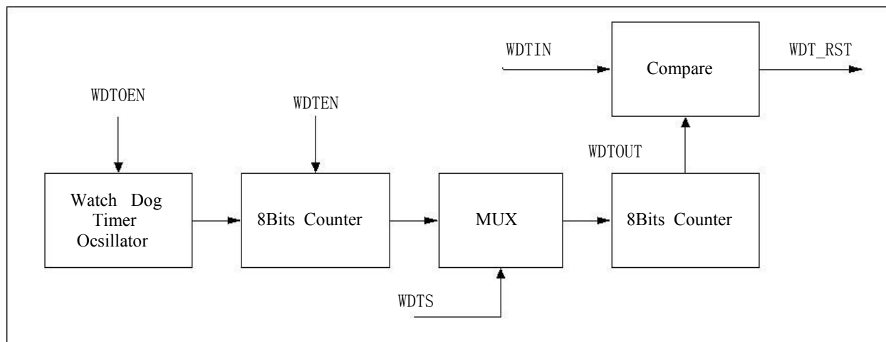
图11 看门狗定时器功能框图
