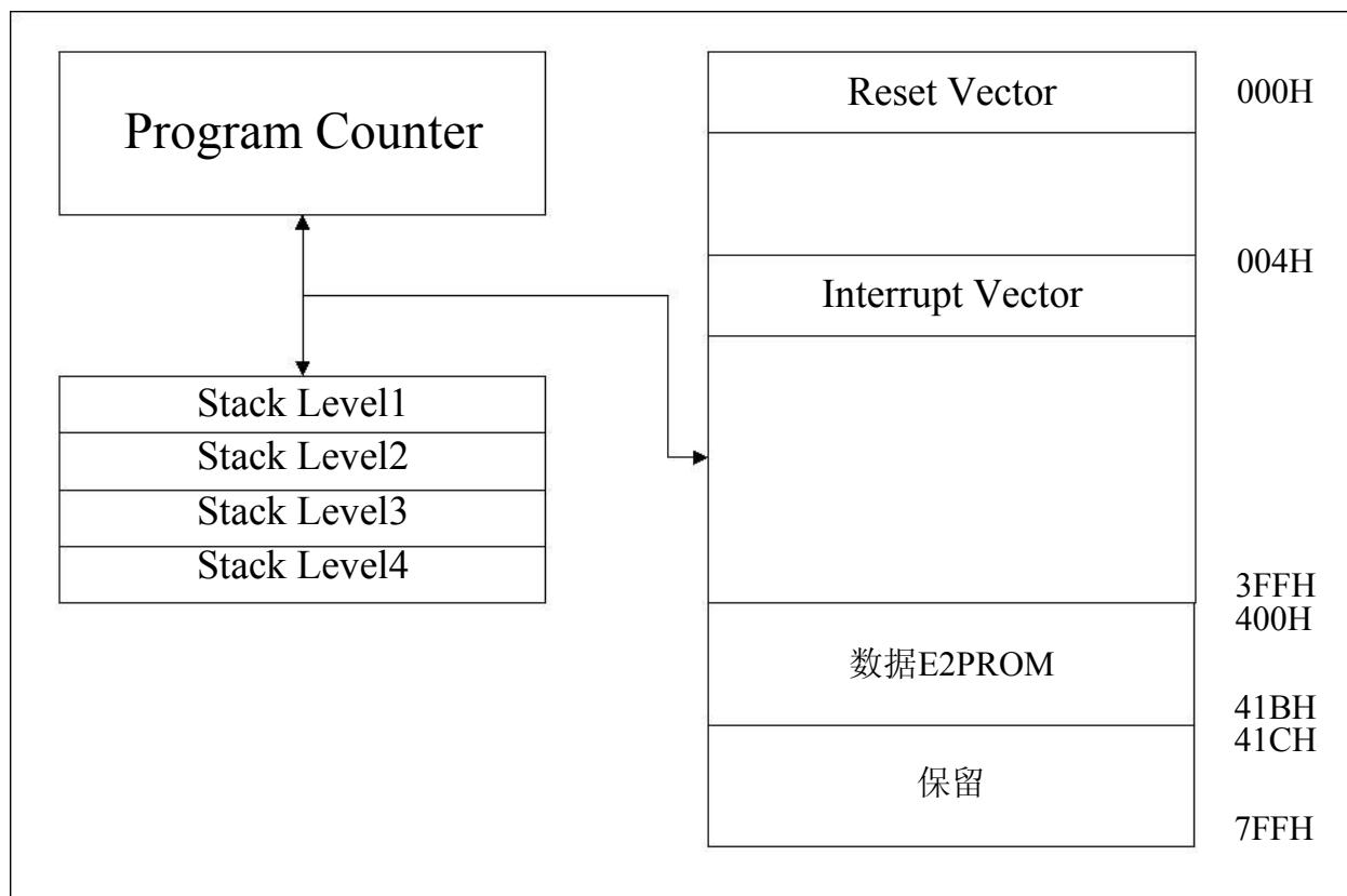
图3 程序存储器
