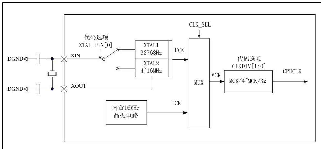
图5 CSU8RF2111/CSU8RF2112振荡器状态框图
