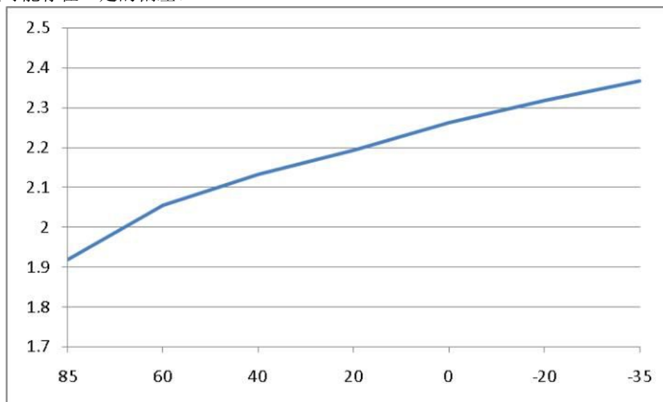
图 11上电复位电压值随温度变化曲线
