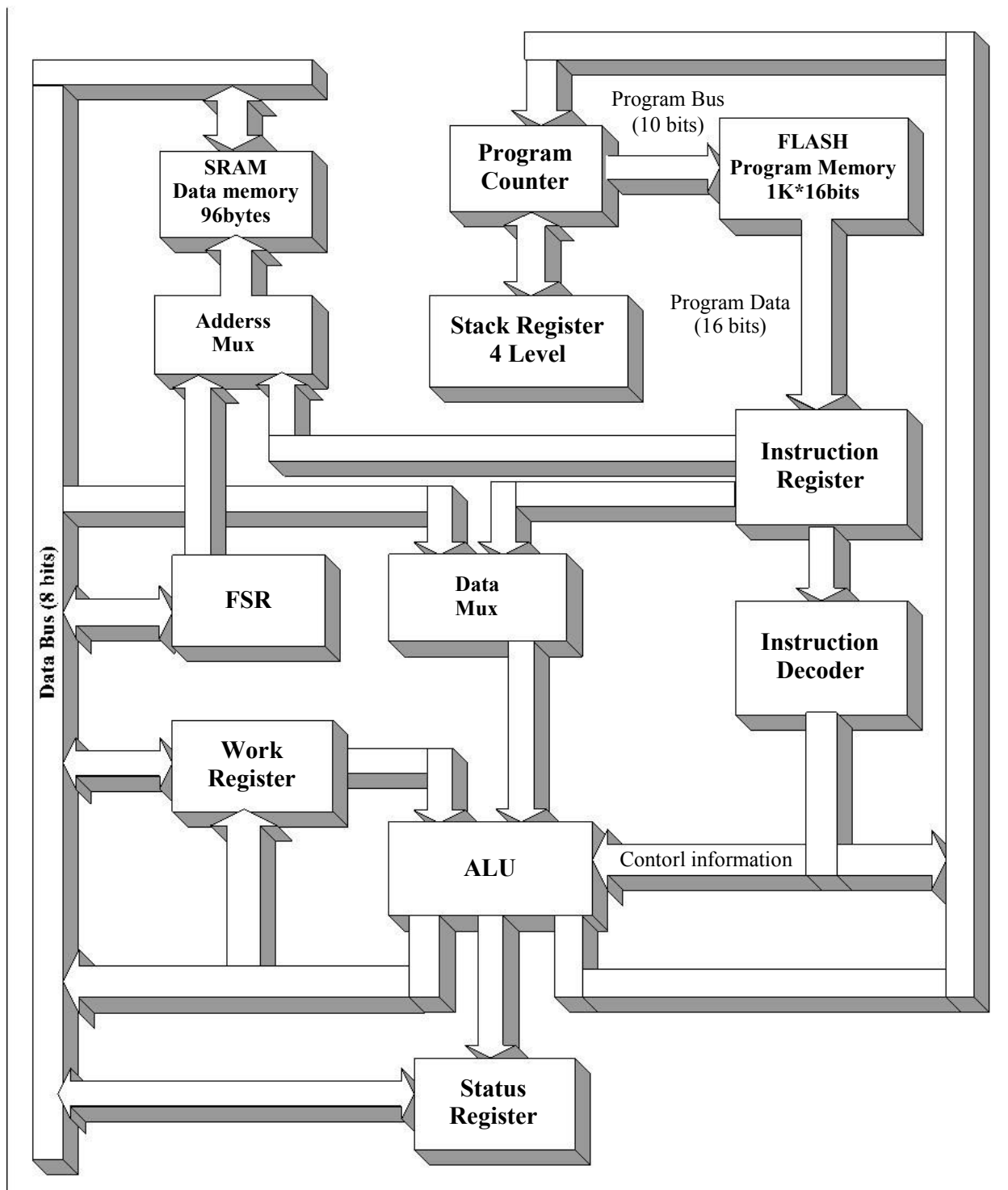
图2 CSU8RF2111/CSU8RF2112 CPU核的功能模块图
