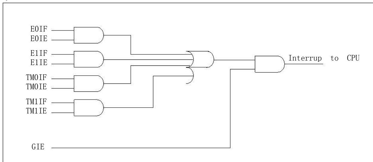
图8 中断逻辑
